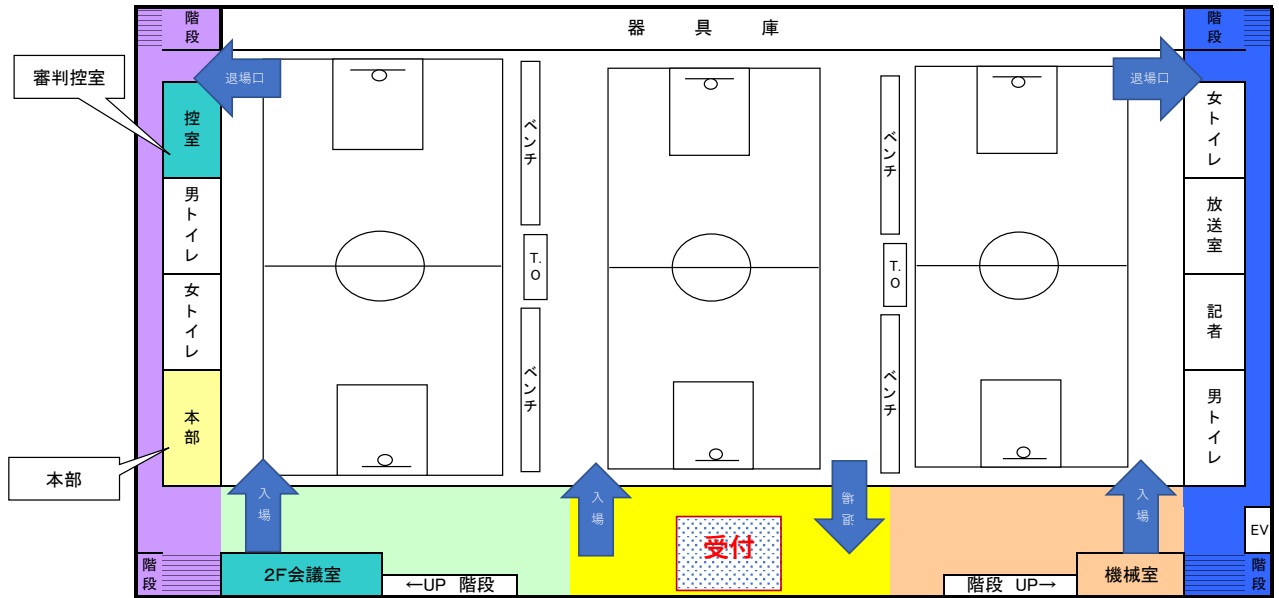
2階平面図
